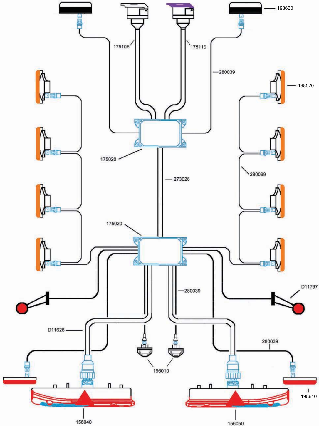
Exemple de montage - Assembly suggestion - Montagebeispiel
