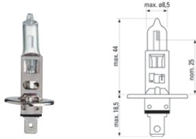
H1 - P14,5s
