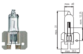
H2 - H511
