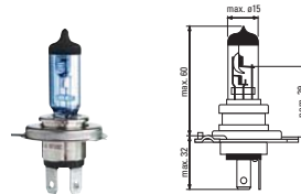
H4 - P43t
