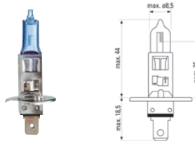
H1 - P14,5s
