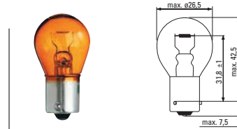
PY21W - BAU15s
