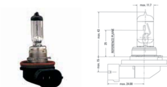
H8 - PGJ19-1
