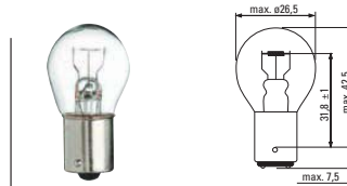
P21W - BA15d
