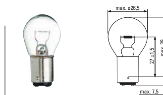
Sphérique - BA15d
