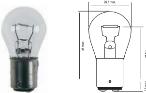
Poirette - BA15d
