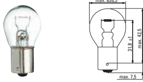
P21W - BA15s
