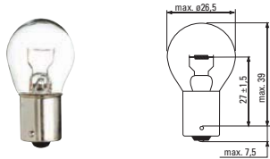
Sphérique - BA15s
