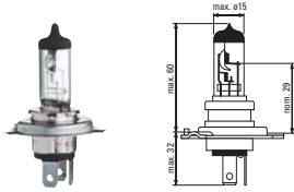
H4 - P43t
