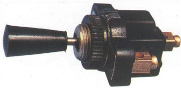
Toggle Switch Merit Type Left - Right Move Code Nr : E0415B
