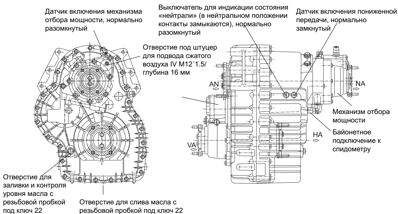
Рис 8: Отбор мощности от раздаточной коробки ESC-166
