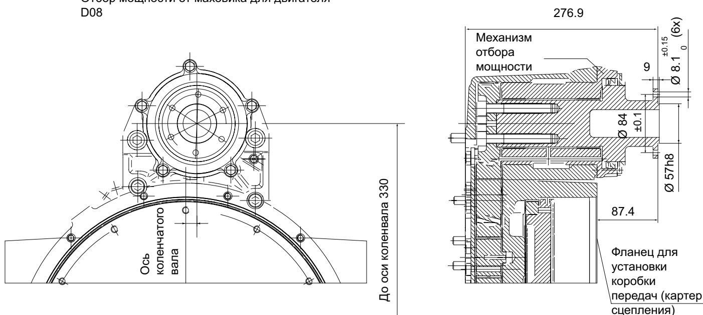
Рис 7: Технические данные механизма отбора мощности у 6-цилиндрового двигателя D08 ESC-830
