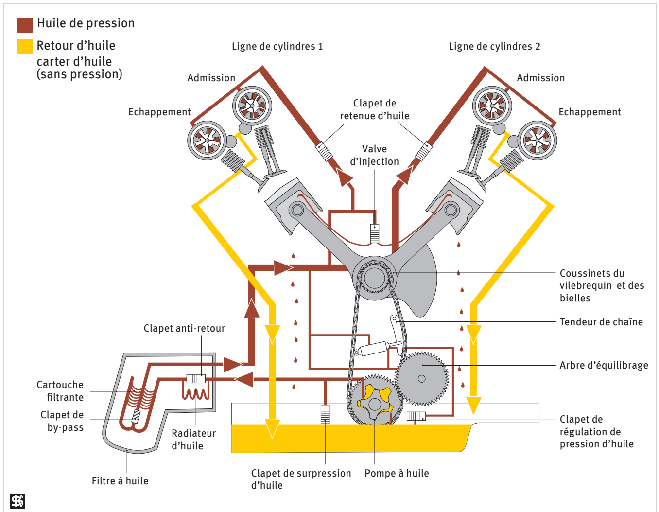
Circulation d'huile
