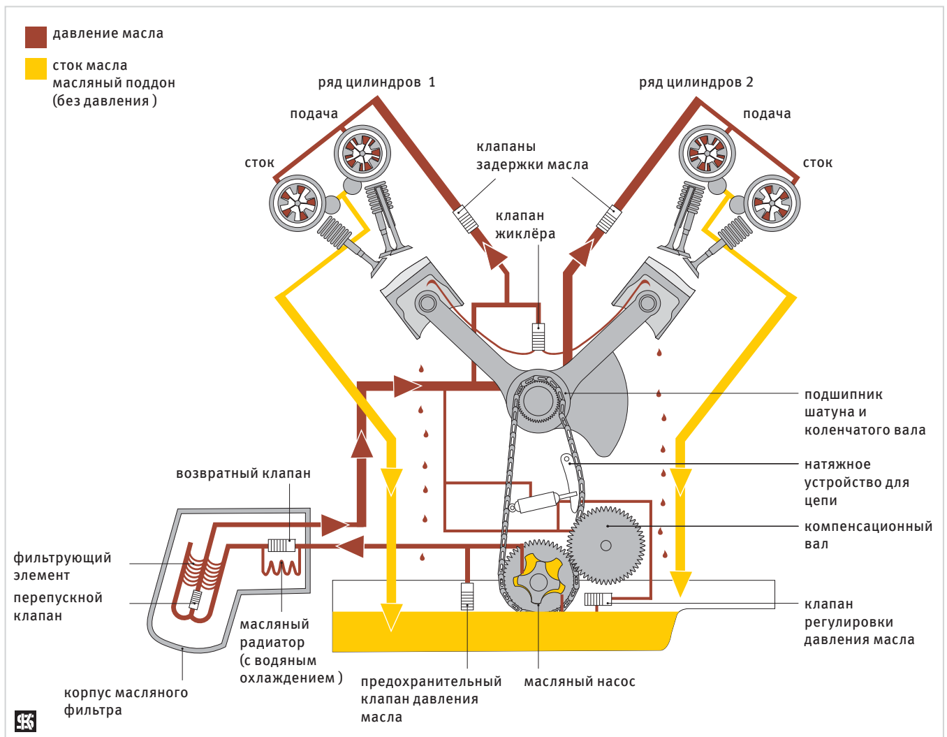
Циркуляция масла
