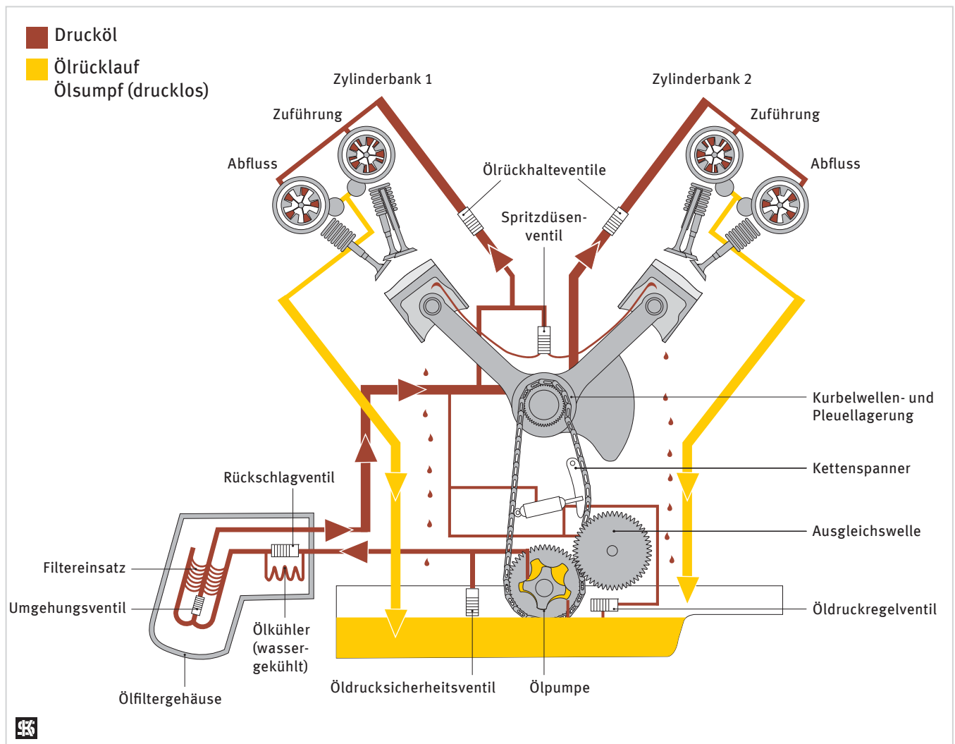
Ölkreislauf
