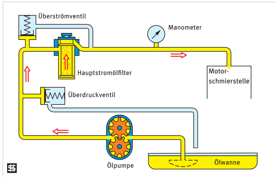
Druckumlaufschmierung
