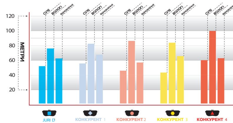
Сухий тест: Тестова швидкість 80 км/год - 0 км/год з 30 зупинками. Вологий тест: 10-хвилинне замочування, в середньому 6 зупинок. Тільки передні гальма.
