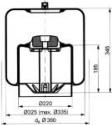
Schnittansicht Cross section view Vue en coupe
