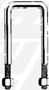
18 - 722020 \varnothing 16x70x250 19 - 722021 \varnothing 16x70x270 20 - 722574 \varnothing 16x70x280 21 - 722022 \varnothing 16x70x300 22 - 722576 \varnothing 16x70x330 23 - 722577 \varnothing 16x70x350 24 - 722578 \varnothing 16x70x370
