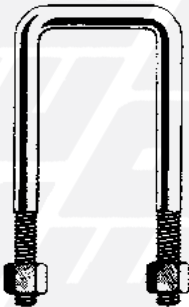
20 - 722061 \varnothing 20x90x160 21 - 722063 \varnothing 20x90x180 22 - 722064 \varnothing 20x90x200 23 - 722065 \varnothing 20x90x220 24 - 722067 \varnothing 20x90x230 25 - 722066 \varnothing 20x90x240 26 - 722068 \varnothing 20x90x260
