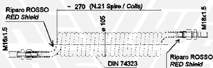
14 - 711808 NERO con RIPARI ROSSI/BLACK with RED SHIELDS
