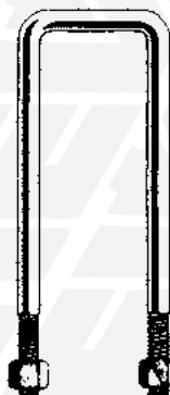
13 - 722574 \varnothing 16x70x280 14 - 722022 \varnothing 16x70x300 15 - 722576 \varnothing 16x70x330 16 - 722577 \varnothing 16x70x350
