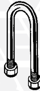
10 723818 \phi 22x130x310 11 723817 \phi 22x130x330 12 723914 \phi 22x130x370
