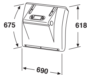
B TGX/516 d/s-rh/lh rechts/links
